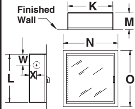
TRIMLESS
